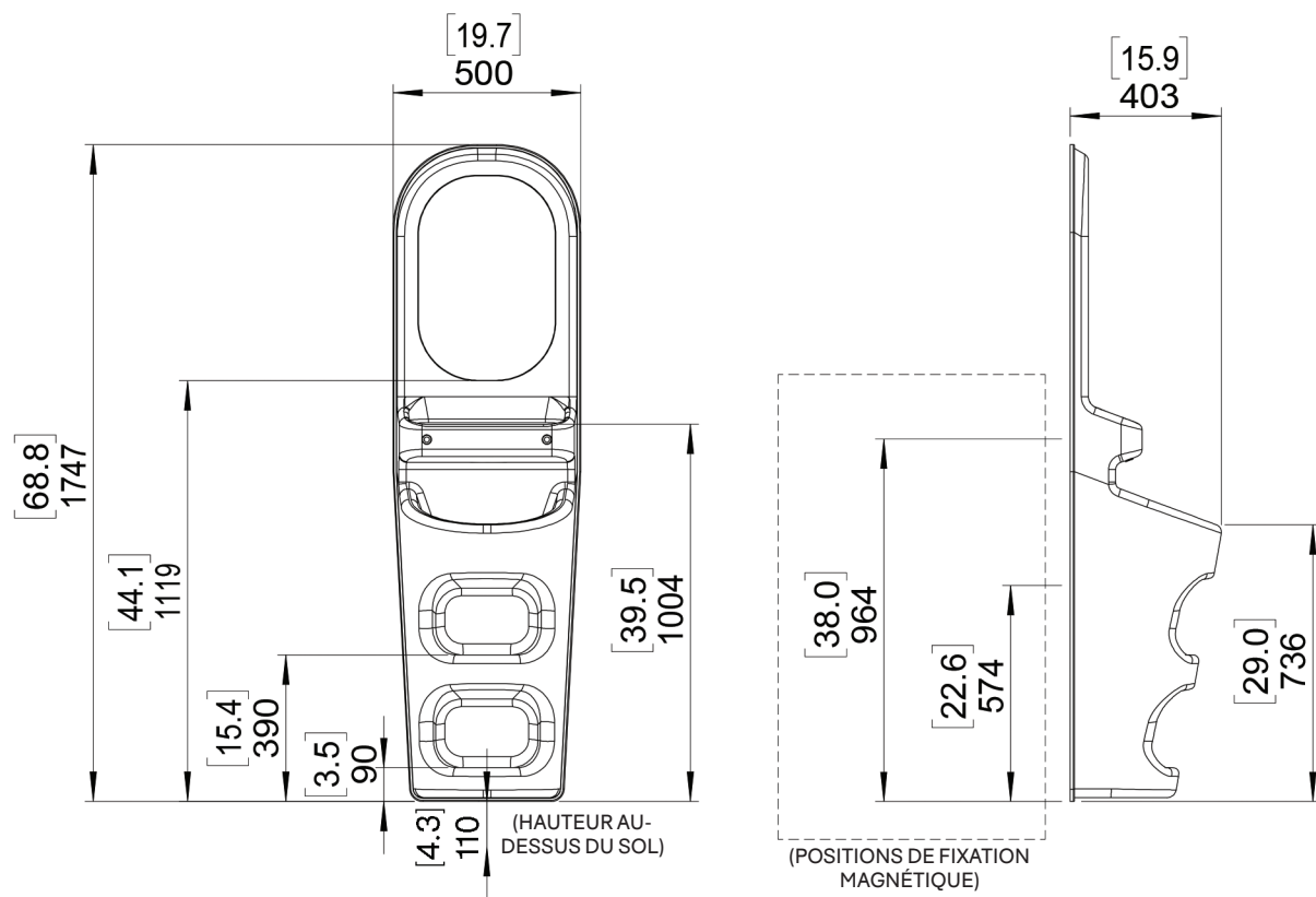
Arc lave-mains avec rangement
